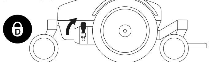
Figure 2. Fonctionnement du levier d'embrayage manuel
