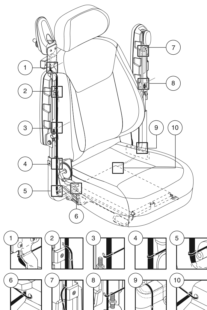
Figure 12. Support d'ancrage système transport
