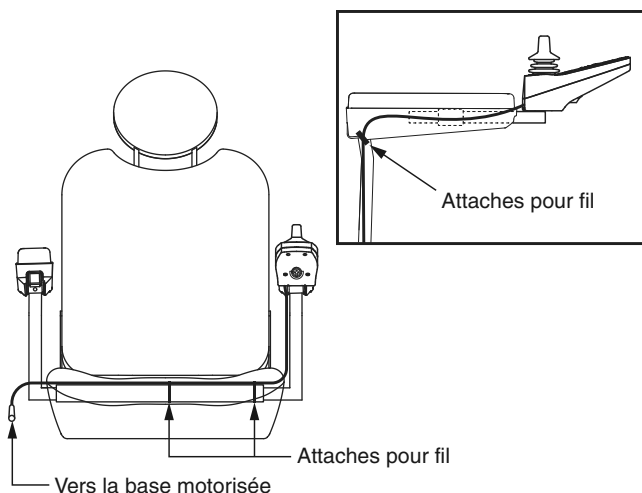
Figure 8. Câble sécurisé sur un siège Contour
