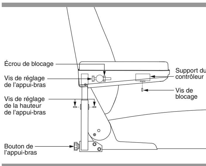
Figure 16. Réglages des appuis-bras et dossier
