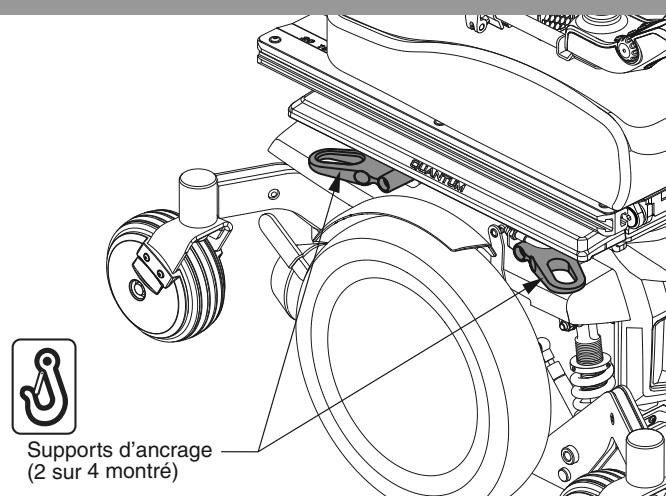
Figure 12. Support d'ancrage système transport
