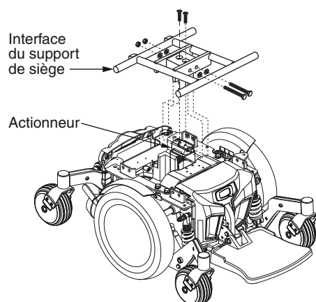
Figure 11. Actionneur du siège électrique élévateur
