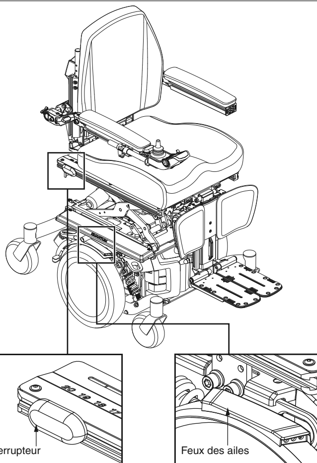
Figure 4. Interrupteur simple pour allumer les feux des ailes
