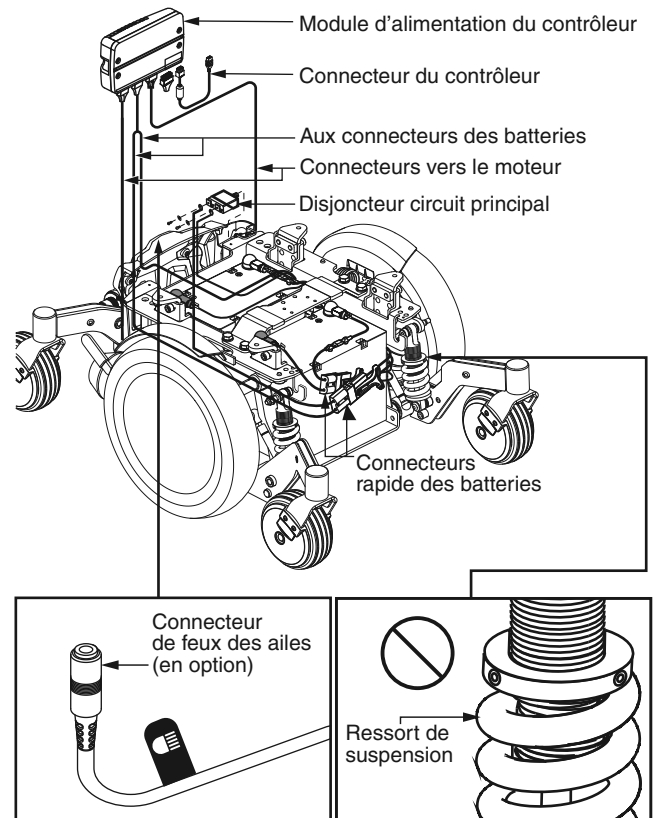
Figure 1. Composantes électroniques
