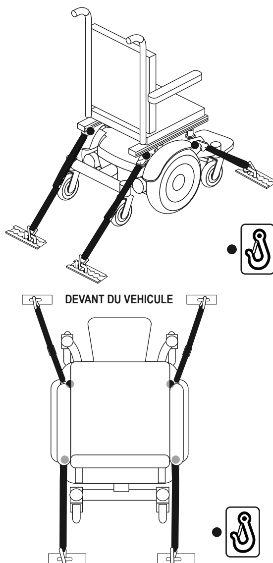
Figure 13. Points d'ancrage pour fauteuil motorisé non occupé
